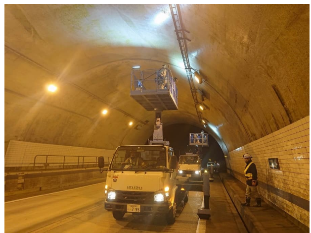
作業状況写真例
