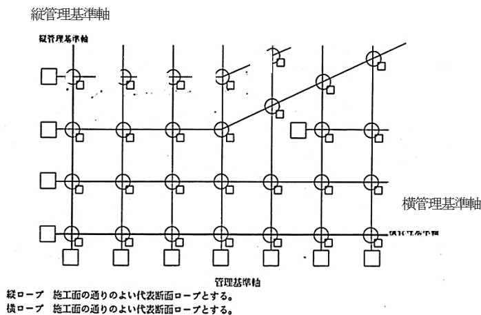
縦・横ロープの基準軸及びロープ間隔の割り付け
