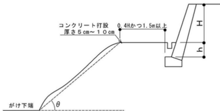
図4-2-5 <擁壁前面がのり面等の場合>
