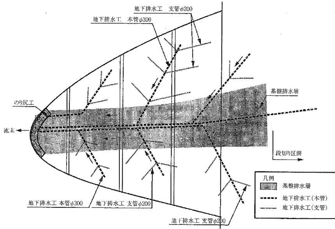
図6-4-4 <盛土内の暗渠排水工及び基礎排水層の設置例>
