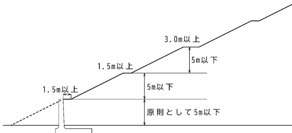
図 3-4-2 <一段目ののり面を擁壁で覆う場合>
