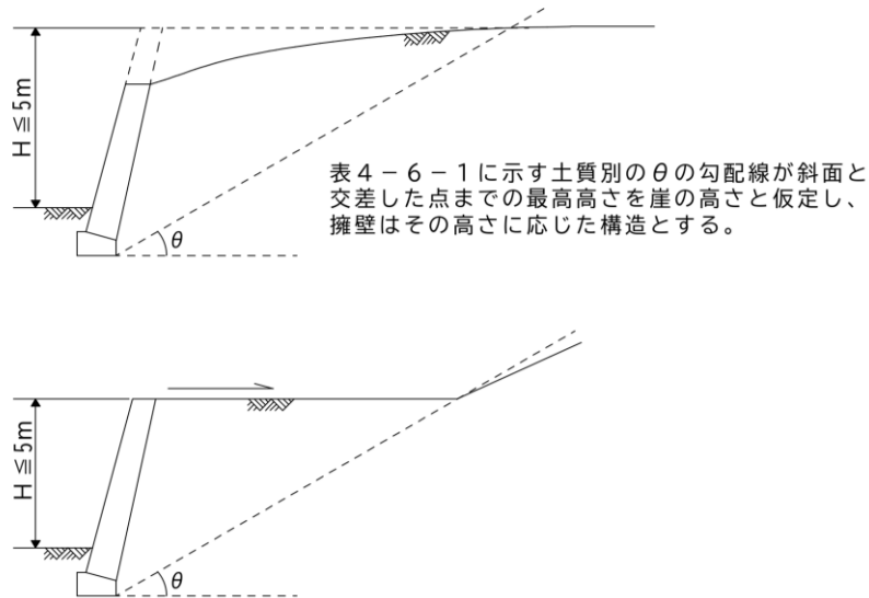
図4-6-1 <切土部分に設ける練積み造擁壁の場合>
