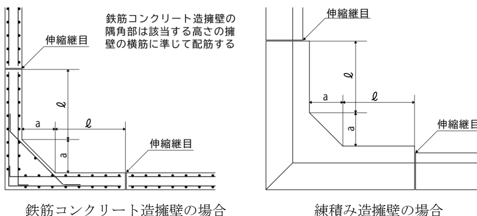
(a) 平面図
