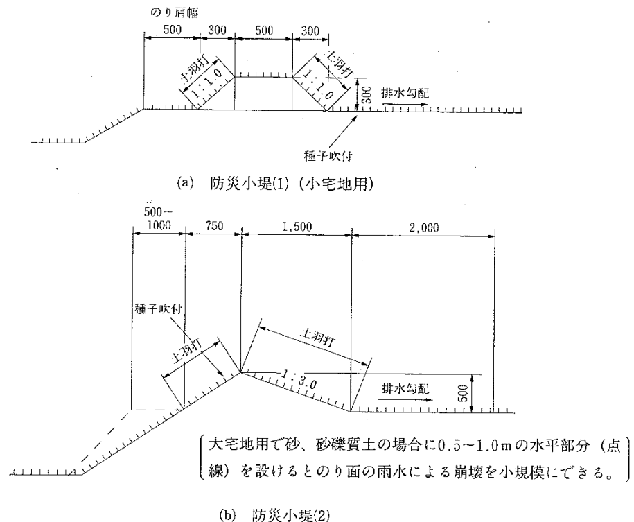
図9-1-1 <防災小堤の形状>
