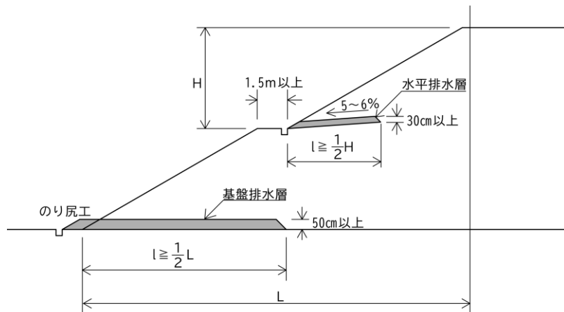
図6-4-5 <基礎排水層及び水平排水層の例>
