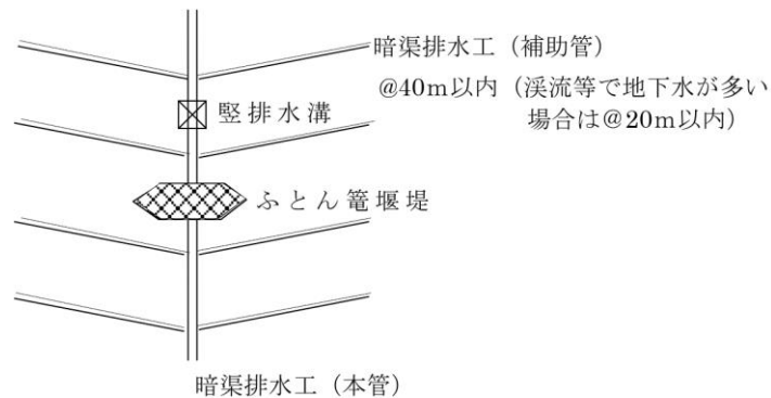
図 6-4-7 <ふとん籠堰堤の例>
