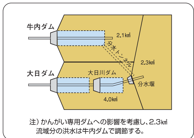
両ダムの洪水著説概要図
