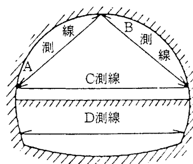
パターンD, E, 坑口附近, 土被の浅い区間, 計測Bを実施する箇所
