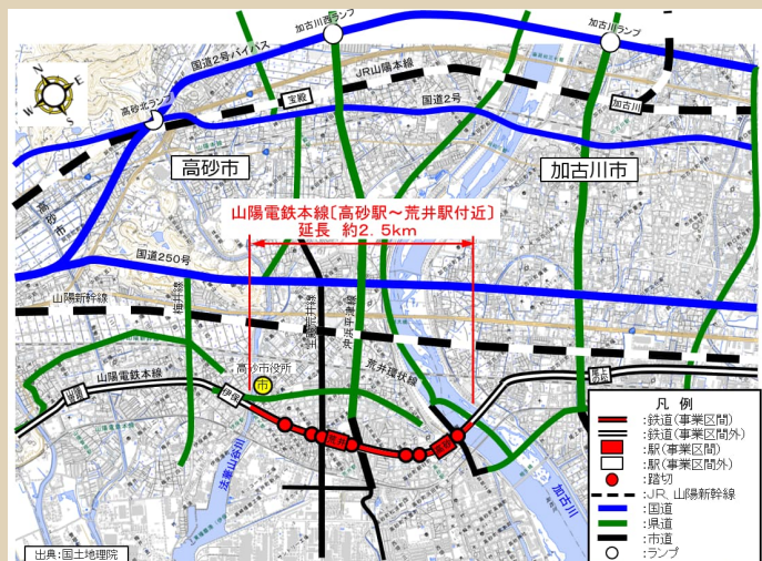
山陽電鉄本線 高砂駅～荒井駅付近 連続立体交差事業
