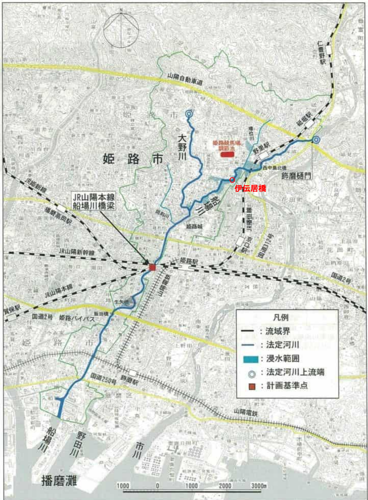
図 1.16 平成 16 年 10 月台風 23 号による実績浸水区域図
