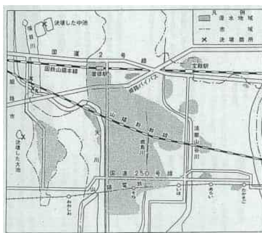
図 1.11 昭和 51 年 9 月の台風 17 号の浸水による被災地域
