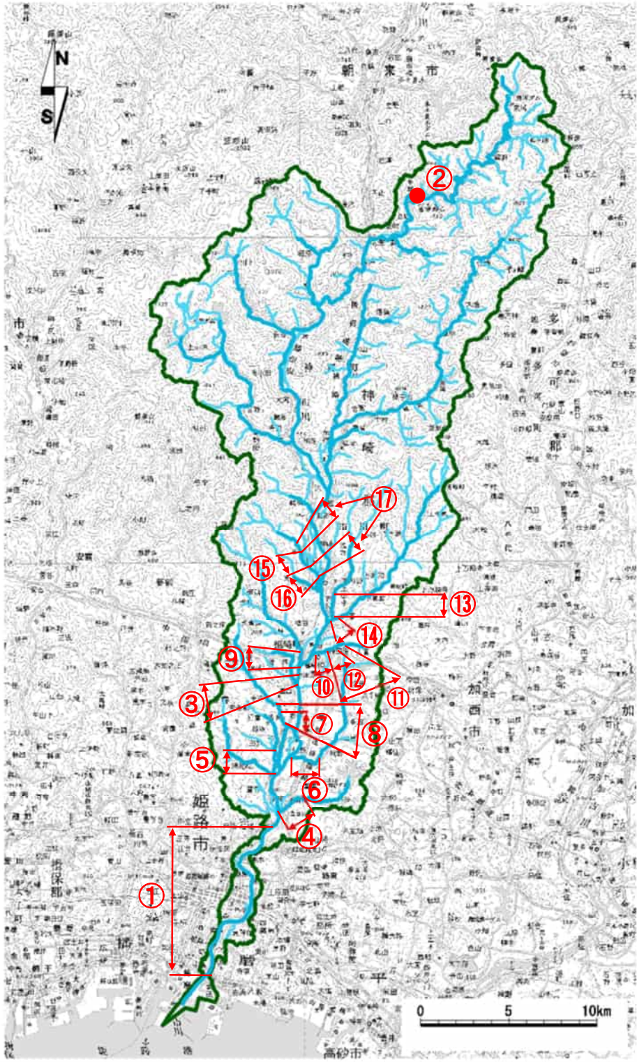
图 1.22 市川水系 治水事業位置图
