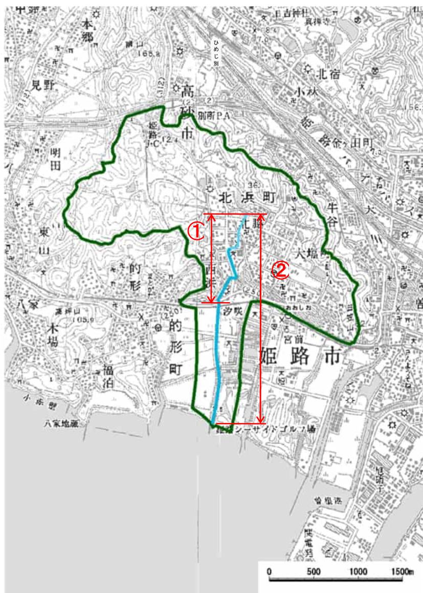
図 1.20 西浜川水系 治水事業位置図
