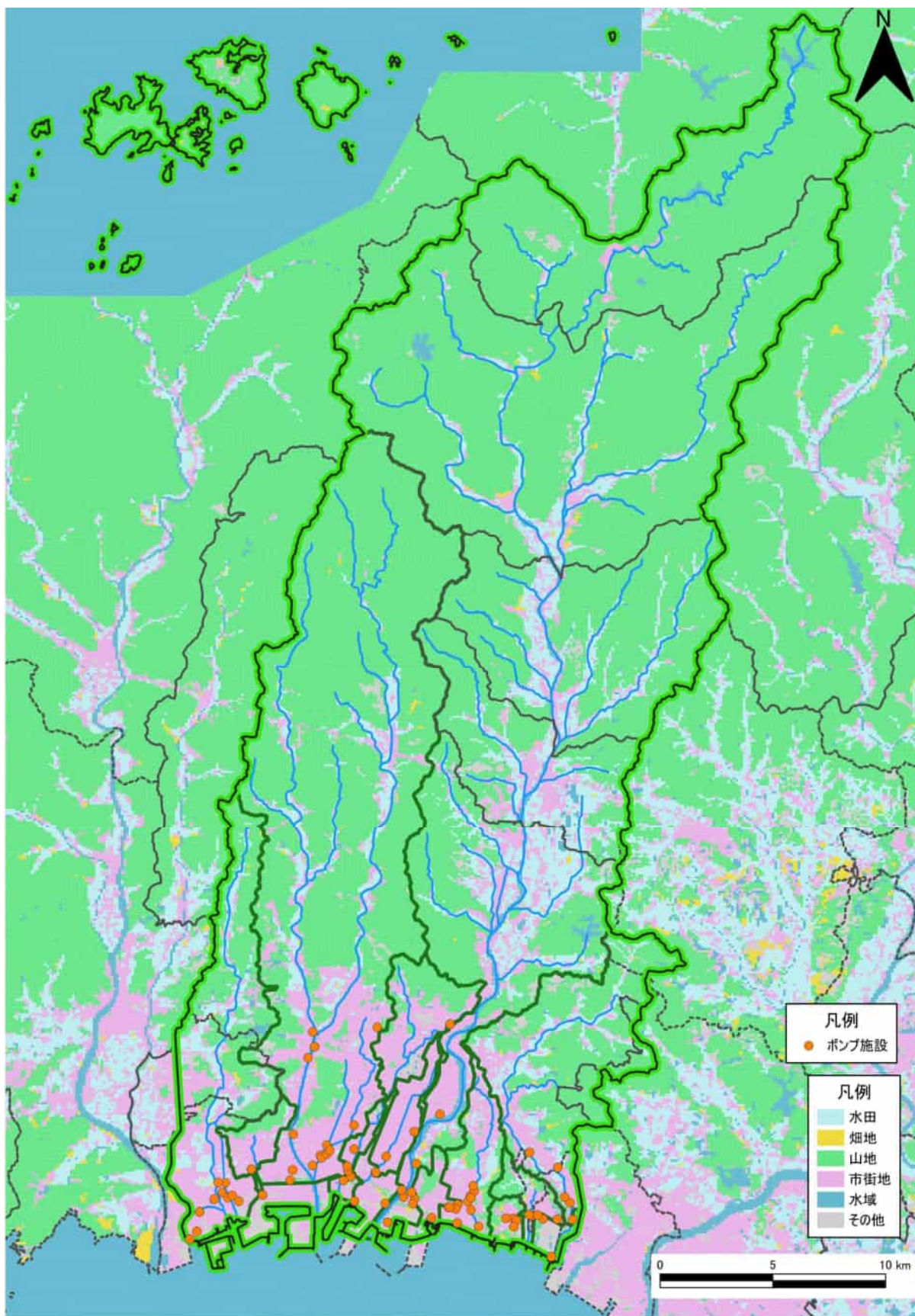
図 2.7 ポンプ施設位置図
