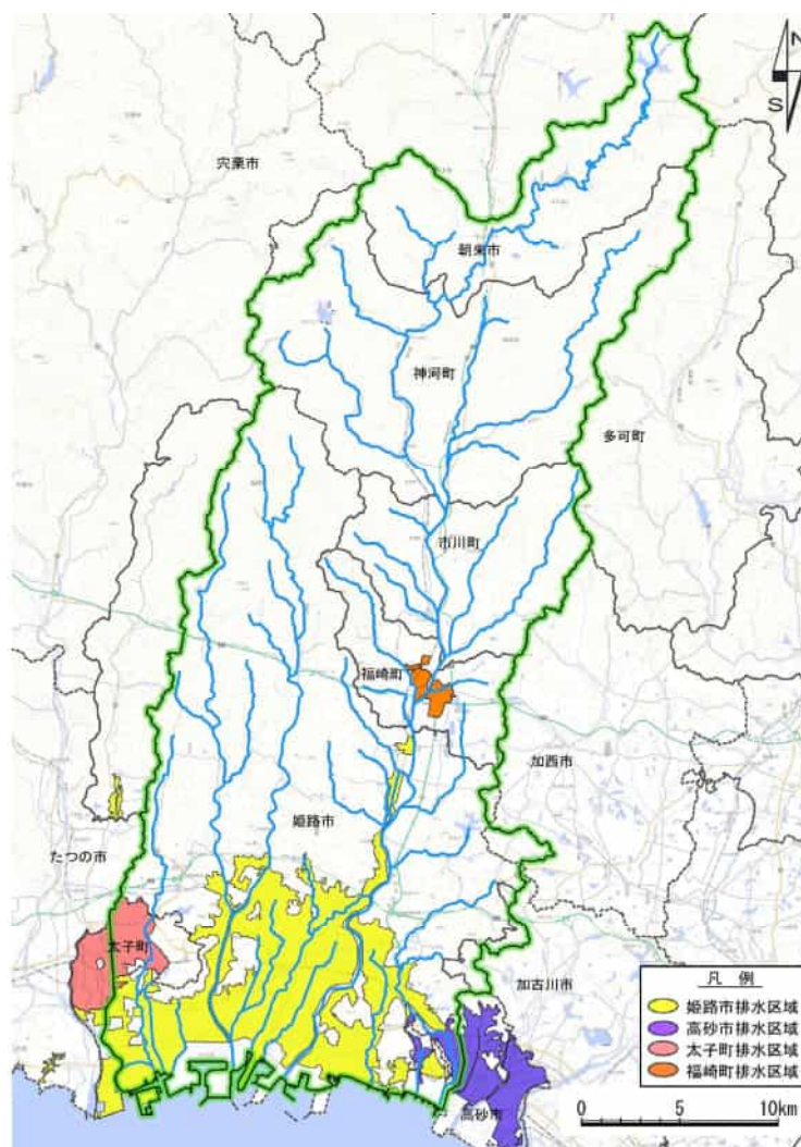
図 1.28 下水道（雨水）区域位置図
