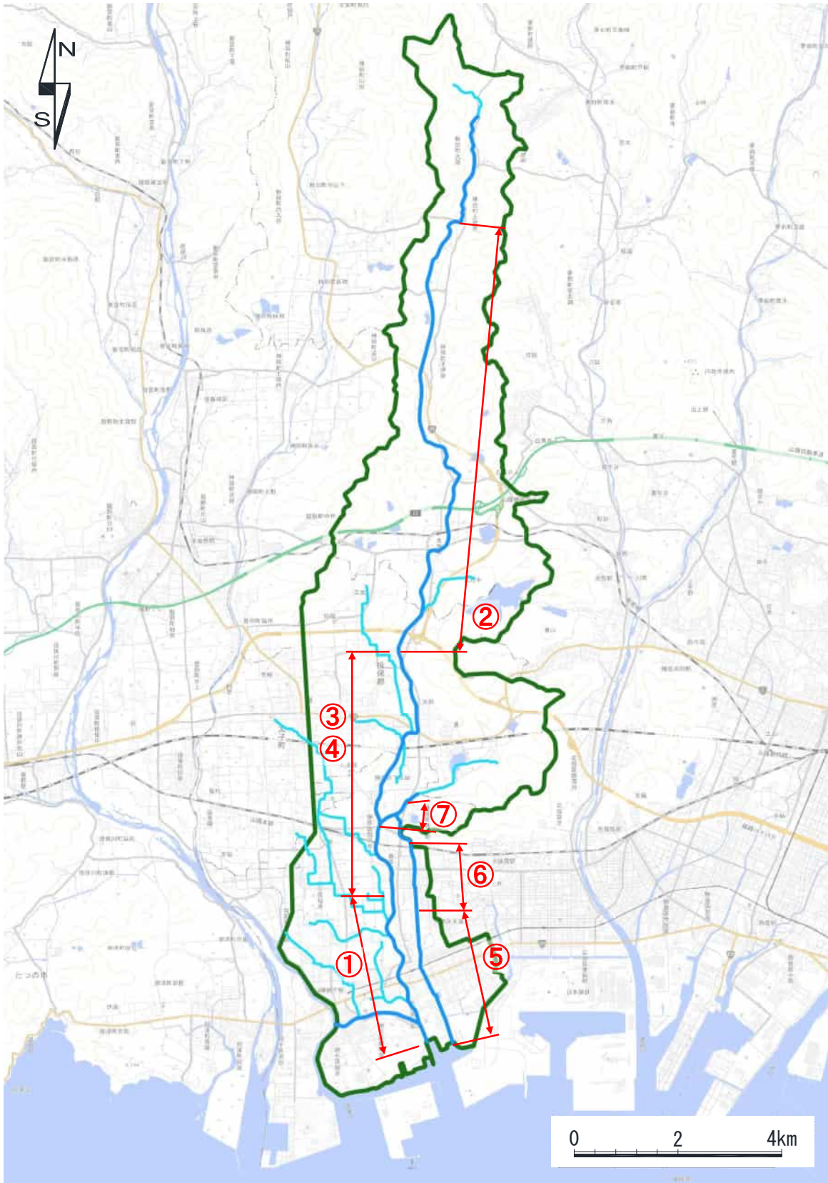
図 1.27 大津茂川水系 治水事業位置図
